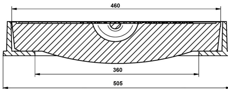
SCHNITT A-A
