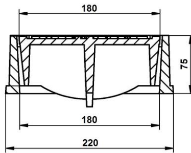
SCHNITT B-B
