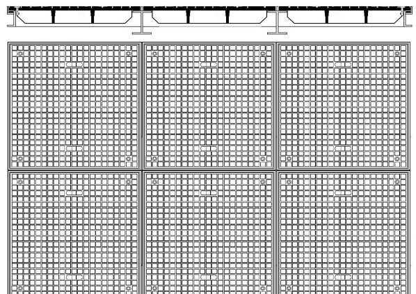
z.B. 6-teilige Flächenabdeckung
