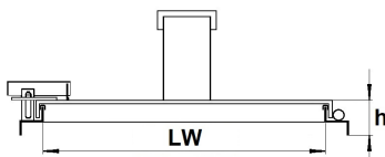
Rahmen zum einbetonieren
